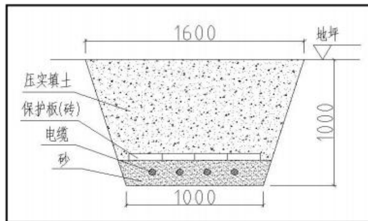
图 2.10-5 直埋电缆典型横剖面图（单位：mm）
