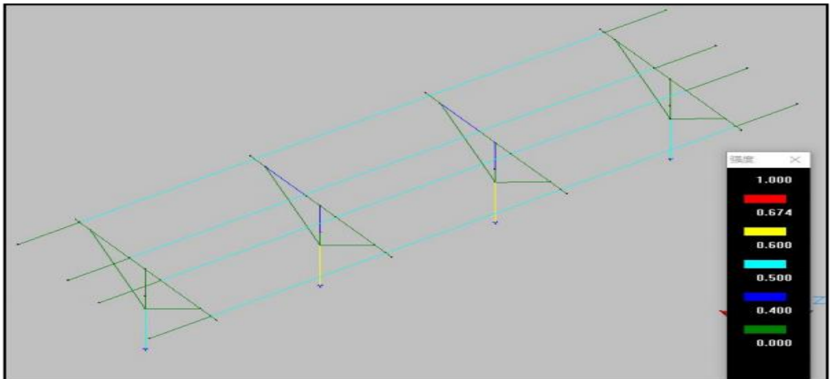
图 2.10-2 光伏支架应力比分布图
