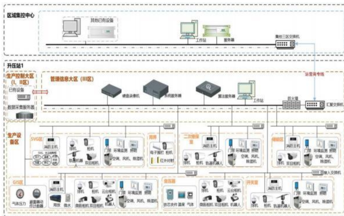
图 2.9-2 网络架构示意图
