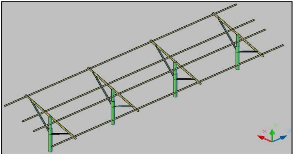
图 2.10-1 光伏支架模型
