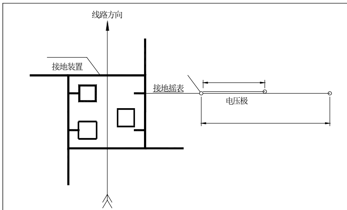
图 2.9-3 接地电阻的测量方法图
